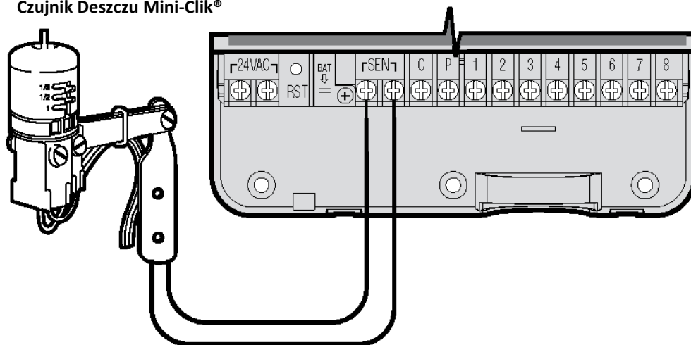
Czujnik Deszczu Mini-Clik®
